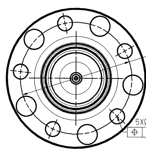
E 向视图
